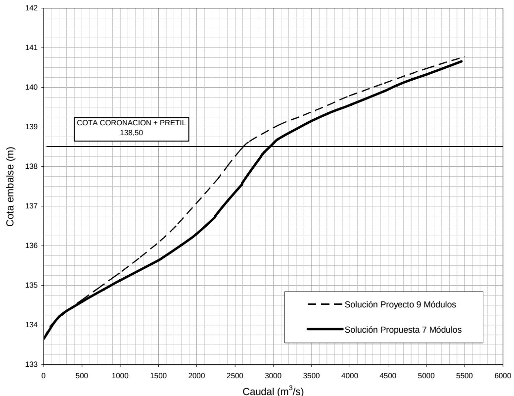
Fig. N° 6. Curvas de capacidad obtenidas experimentalmente
