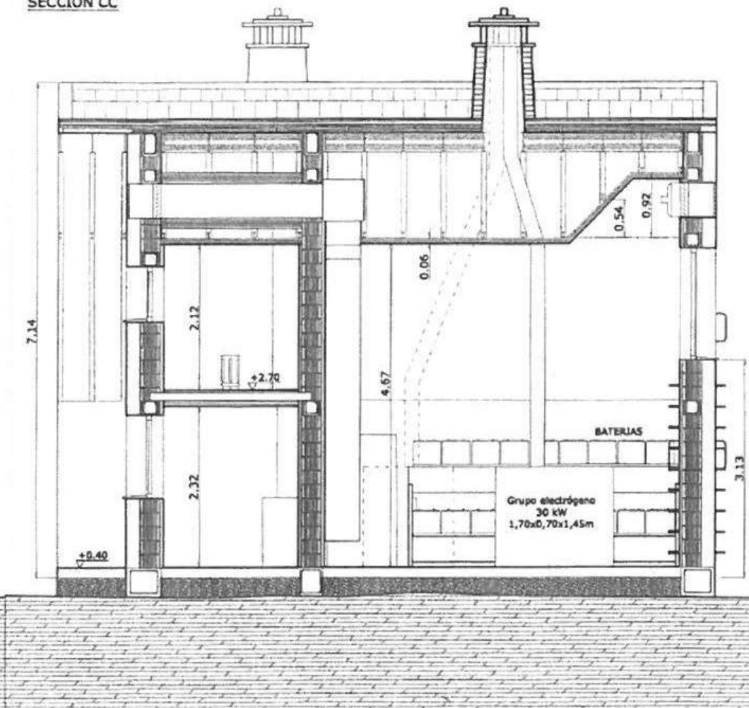
SECCION CC
