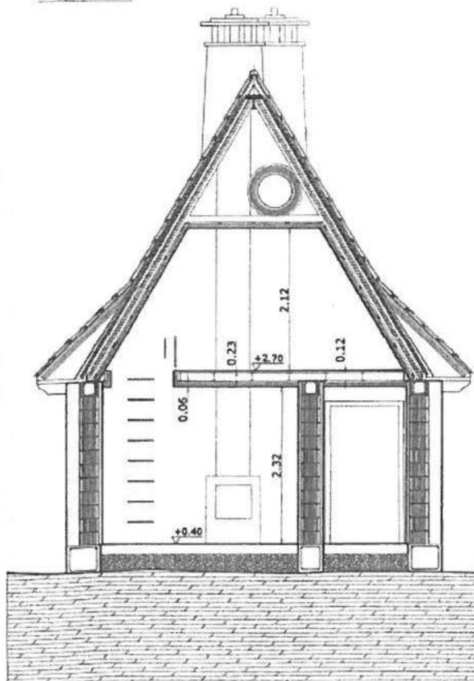
SECCION BB
